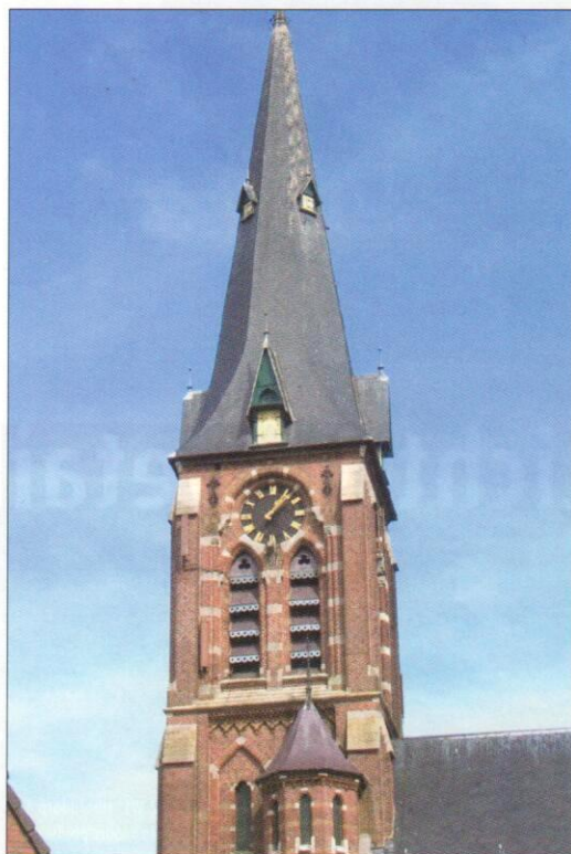
Afb 1. Boven in deze kerk is een antenne-installatie aangebracht en geheel aan het oog onttrokken. Het linker raam in het bovenste galmgat is origineel, het rechter exemplaar (met de antenne) werd gekopieerd.
